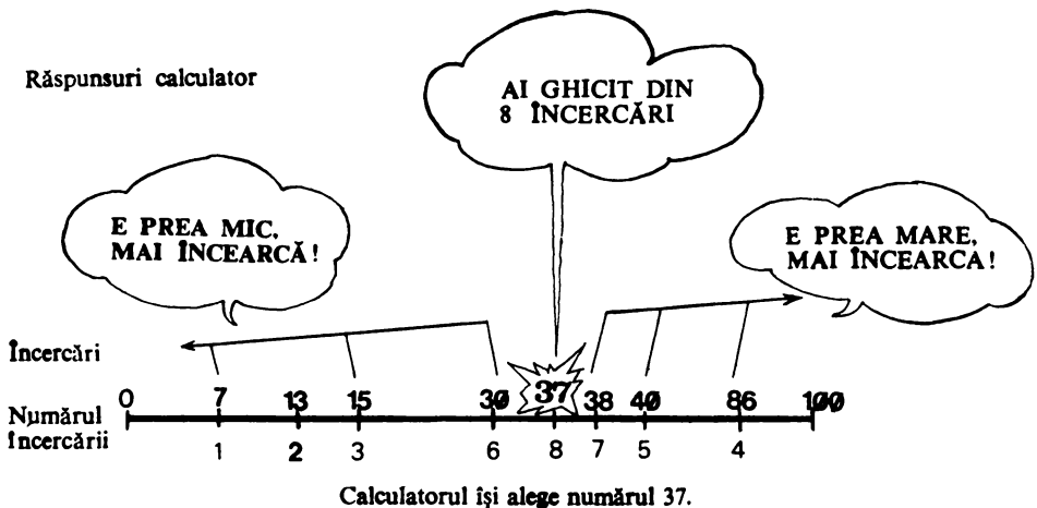
Fig. 27 GHICEȘTE NUMĂRUL
